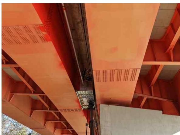
작업전경
